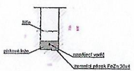
PŘÍKLAD ULOŽENÍ VODIČŮ VE VOLNÉM TERÉNU
