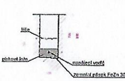
PŘÍKLAD ULOŽENÍ VODIČŮ VE VOLNÉM TERÉNU
