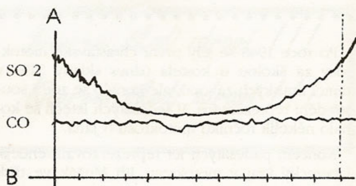
Graf - roční průběh znečištění ovzduší CO a SO 2
